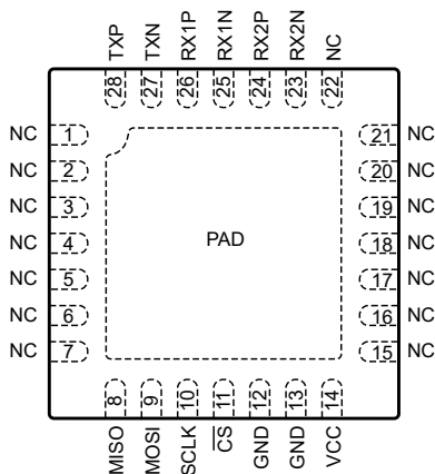
ET Package Pinouts
